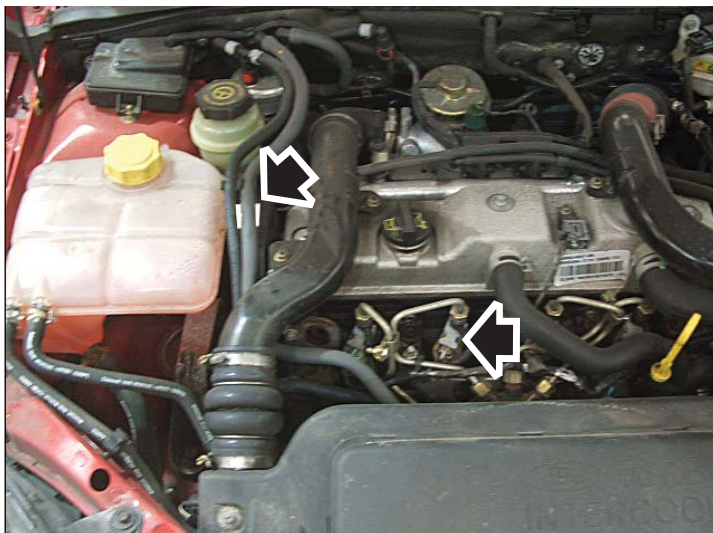
Etiqueta de inyectores y cabeza de inyector indicadas con flechas: Vista frontal
