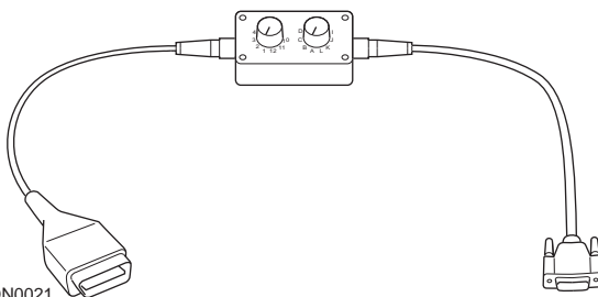
A2C59512073 - Cable múltiple de EOBD
