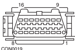
Toma para diagnóstico J1962
